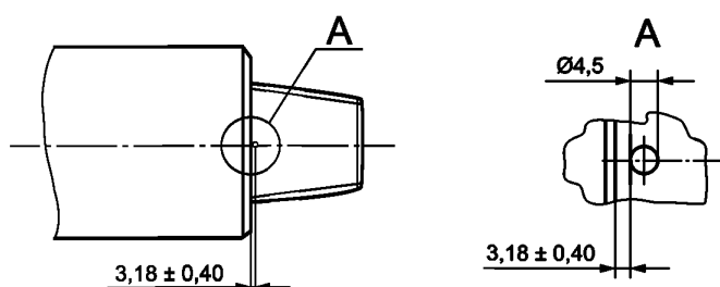
а) Штампованная метка на ниппеле
