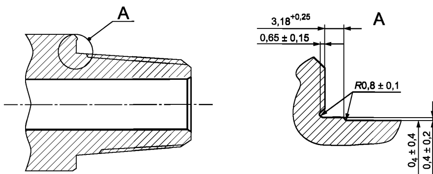
б) Цилиндрическая метка на ниппеле
