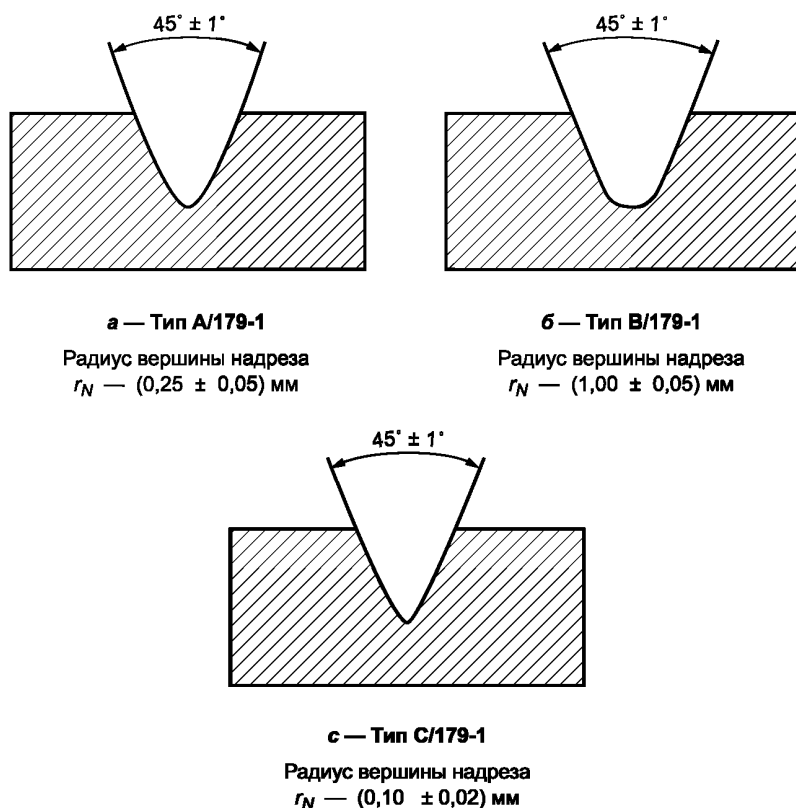
Рисунок 6 — Типы надрезов
