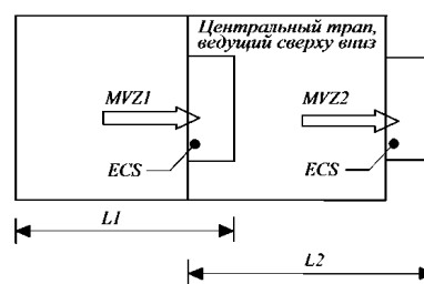
Рис. 2.2.1.2-1 Эвакуационный трап обслуживает одну главную вертикальную зону
