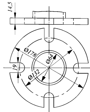
Рис. 5.1.18 Международное береговое соединение (судно)
