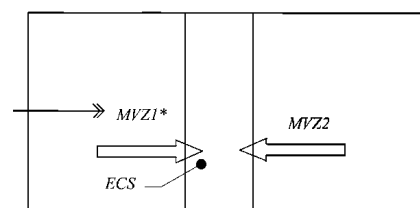
Вариант 1. Эвакуационный трап принадлежит главной вертикальной зоне 1
