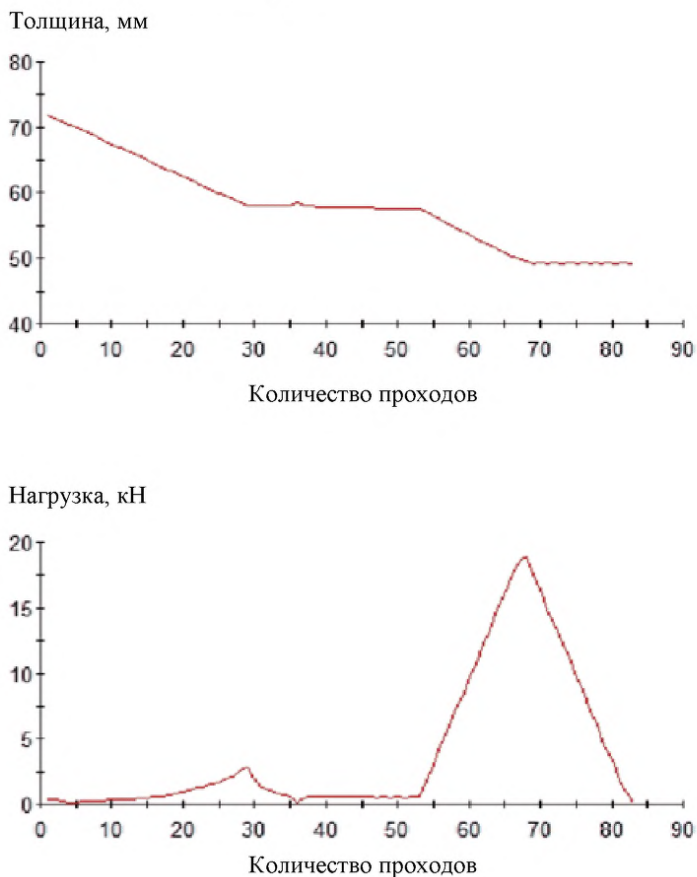
Рисунок 1 – Пример зависимости толщины от количества проходов и нагрузки при уплотнении.
