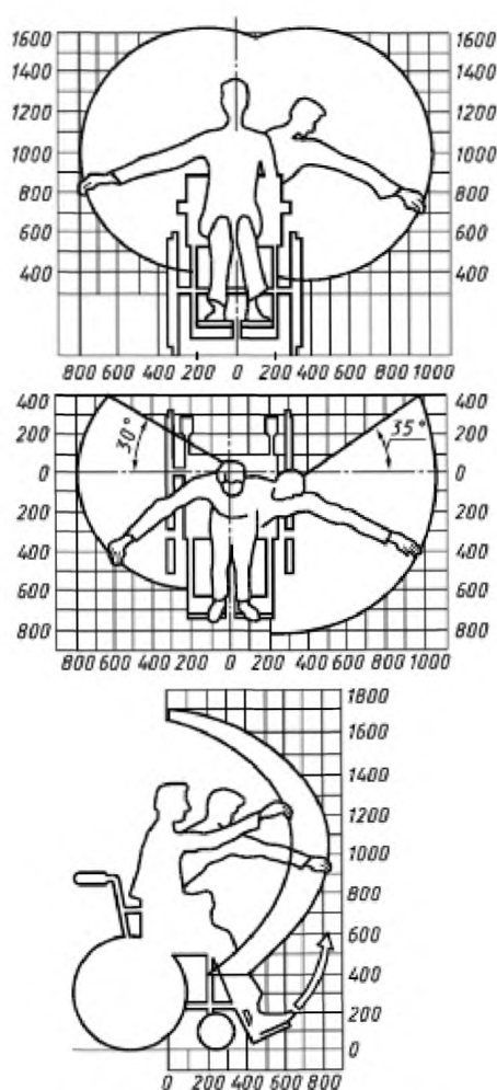
Рисунок 1 — Зоны досягаемости для мужчин в кресле-коляске
