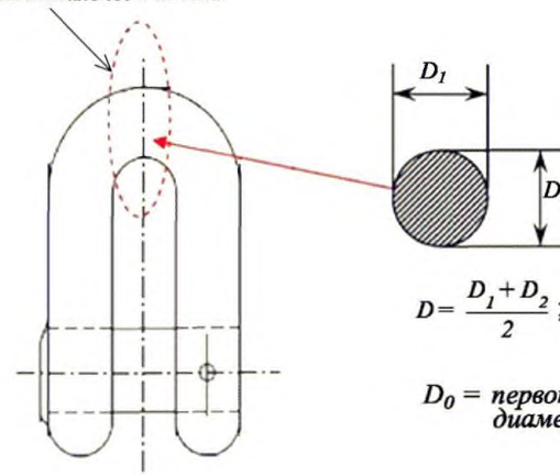
Рис.4. Места замеров скобы (якорной, концевой и соединительной) и максимально допустимый износ
