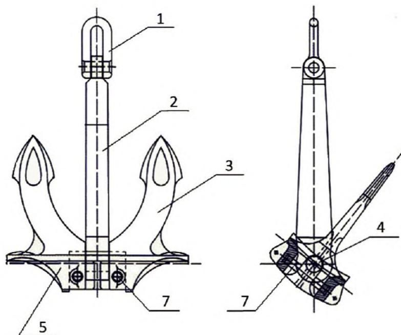
Рис.1 Устройство якоря Холла
