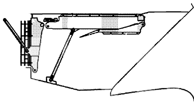
Рис. 2 Носовая грузовая аппарель – положение «по-походному», кормовая часть (внутренняя дверь) отсоединена
