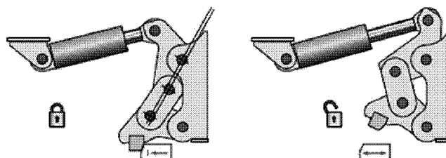
Рис. 17 Клиновая задрайка
