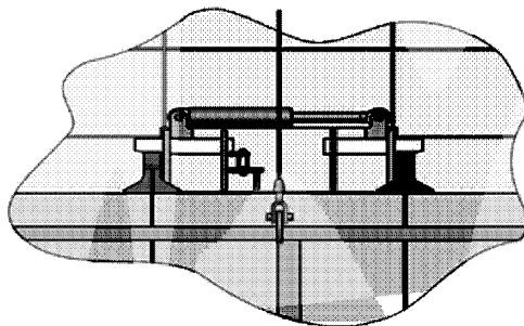
Рис. 31 Грузовая дверь – верхнее боковое гидравлическое закрывающее устройство задрасно
