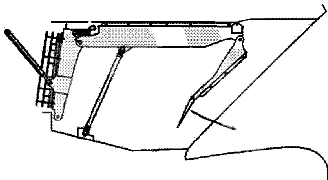
Рис. 3 Носовая грузовая аппарель – начало процесса открывания, кормовая часть (внутренняя дверь) присоединена посредством оси гидравлического шарнира
