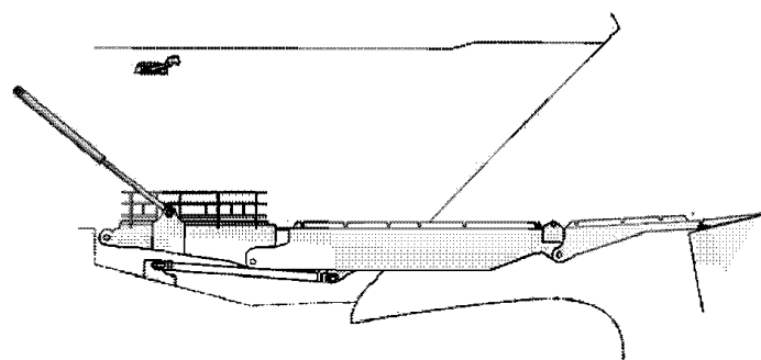
Рис. 4 Носовая грузовая аппарель – аппарель частично выдвинута
