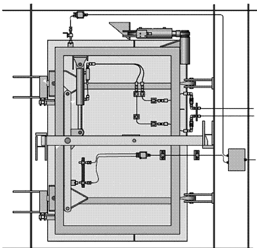
Рис. 36 Лодманская дверь – вид изнутри
