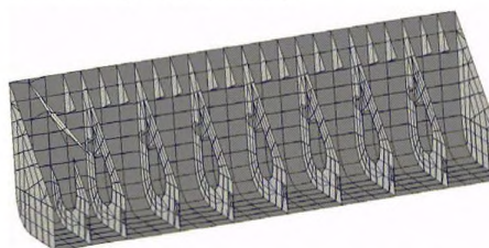
Рис. 2.2.3.2. Скуловые танки
