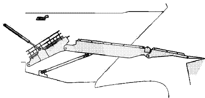
Рис. 3 Носовая грузовая аппарель – начало процесса открывания, кормовая часть (внутренняя дверь) присоединена посредством оси гидравлического шарнира
