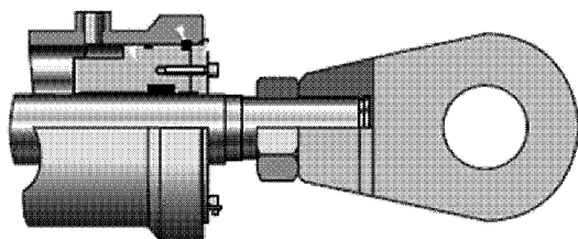
Рис. 19 Гидравлический привод 2
