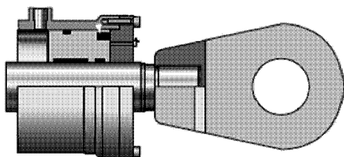
Рис. 20 Гидравлический привод 3
