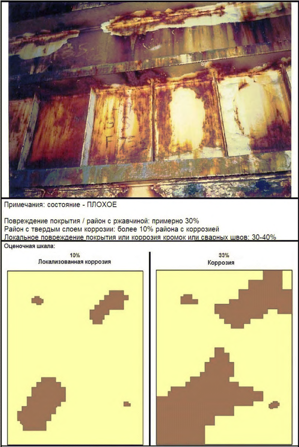
Рис. 2.3.4 - Определение состояния покрытия
