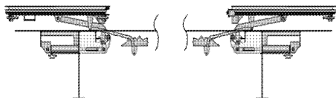
Рис. 34 Бортовая дверь – двухстворчатая, полностью открыта, вид сверху
