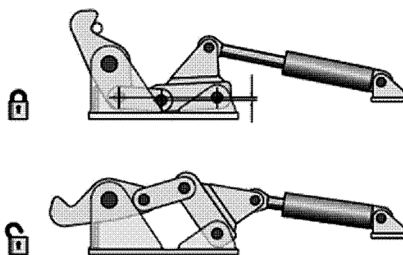
Рис. 16 Стопорный гак 2
