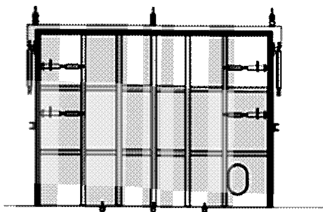
Рис. 2 Носовая грузовая аппарель – положение «по-походному», кормовая часть (внутренняя дверь) отсоединена
