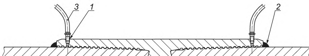
1 — отверстие с резьбовым штуцером на участке муфты, соответствующем сбегу резьбы трубы; 2 — герметизирующий материал; 3 — гибкий шланг
