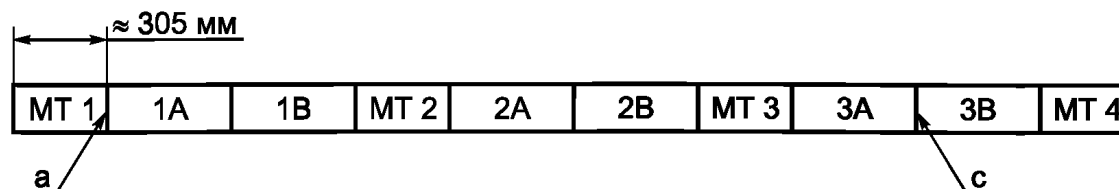
с) Исходная заготовка 1 — длинные патрубки (для механической обработки могут потребоваться более длинные отрезки)
