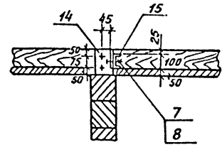
Разрез 5-5
