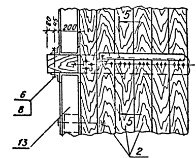
План 3-3
