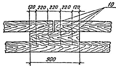
Соединение продольных брусьев
