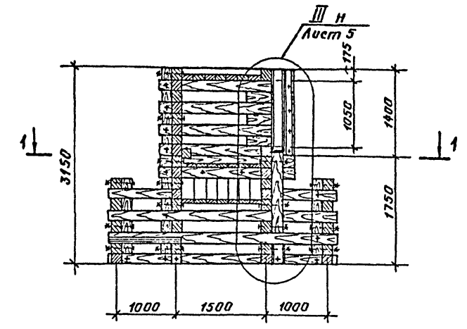
РАЗРЕЗ 3-3
