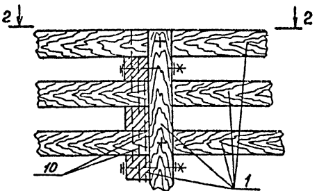
План 2-2
