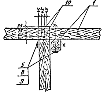
План 2-2
