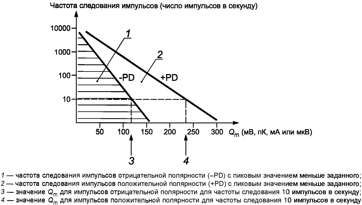
Рисунок 9 — Результаты анализа частичных разрядов
