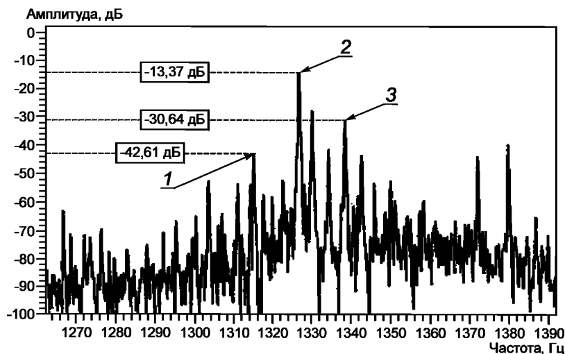
Рисунок 4 — Пример спектра сигнала тока двигателя в случае значительного эксцентриситета воздушного зазора
