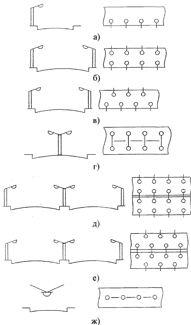
Рисунок 1 – Схемные решения типовых осветительных установок УНО
