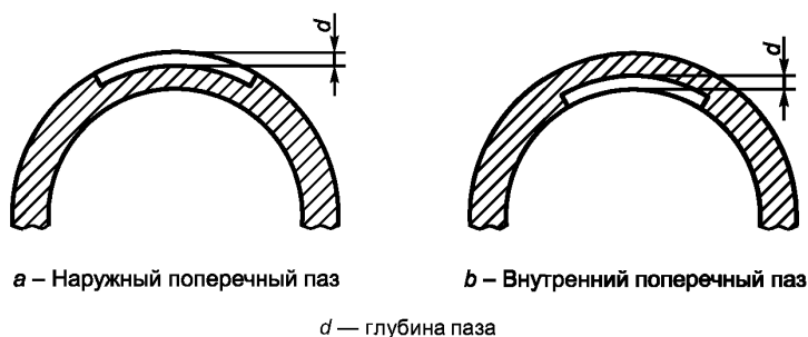
Рисунок 4 — Возможные формы поперечного паза
