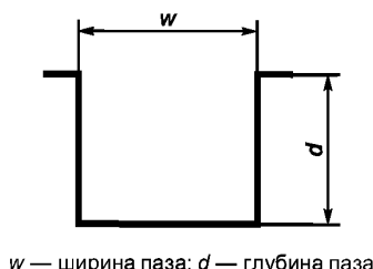
Рисунок 3 — Паз «N»-типа
