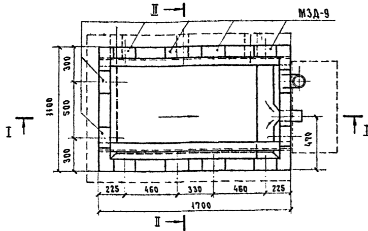
ПЛАН М 1:20 (Крышка не показана)
