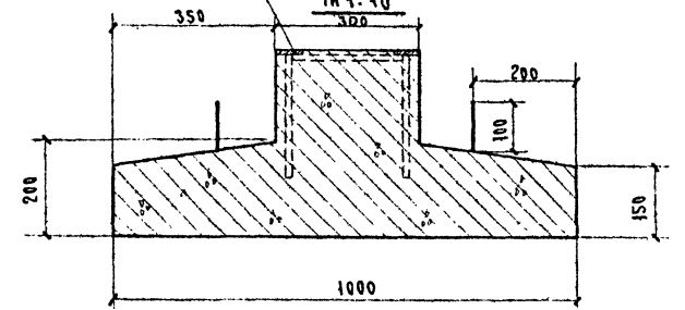
МЗД-1 (МЗД-1°) В-В повернуто М 1:10
