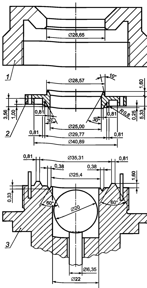
Рисунок 1 — Детали зажима и головки
