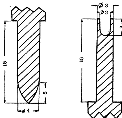
Рис.6. Угольные электроды
