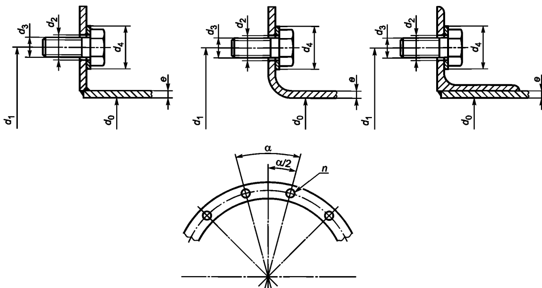
Рисунок 4 — Размеры круглых фланцев
