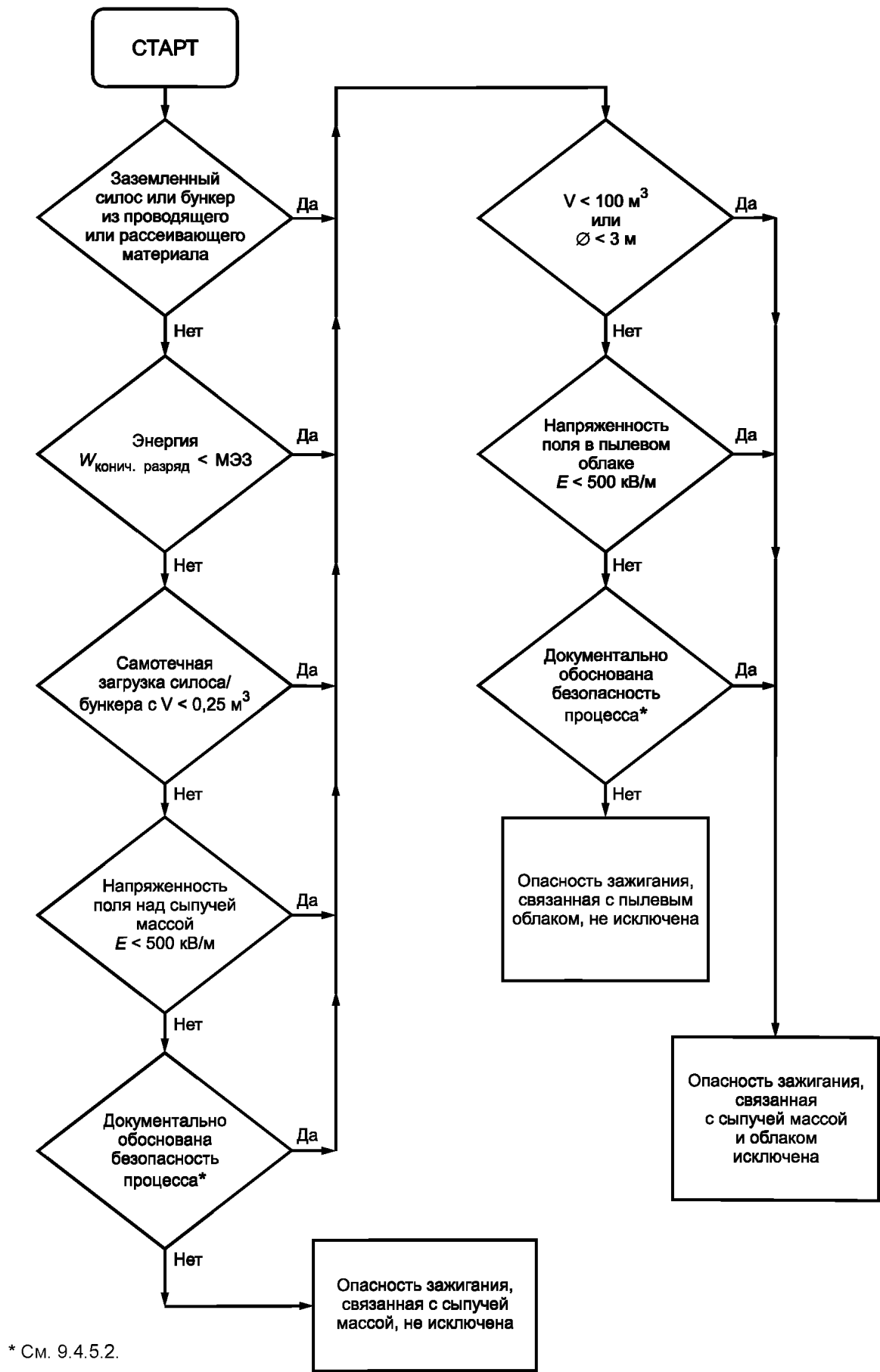
Рисунок 2 — Блок-схема: оценка сыпучего материала с 1 \text{ МОм} \cdot \text{м} < \rho \leq 10 \text{ ГОм} \cdot \text{м}
