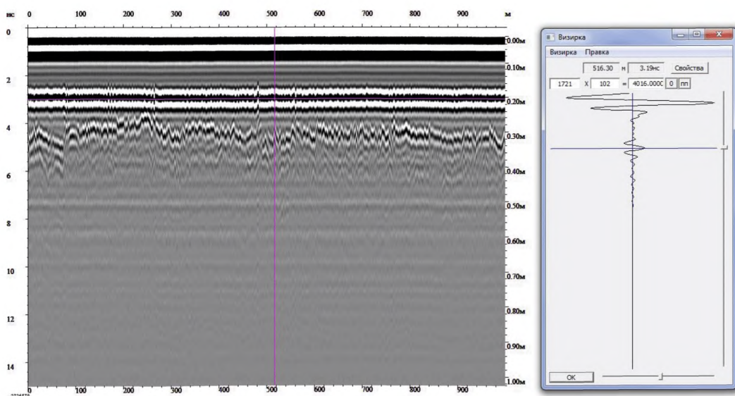
Рисунок Д.1 – Пример смещения вертикальной шкалы глубин
