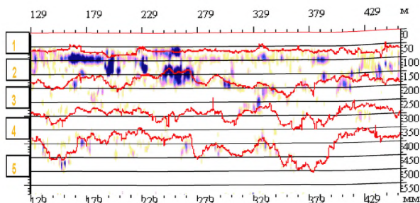
Рисунок 9 – Выделение зон с различной степенью плотности материалов дорожной одежды и грунтов земляного полотна
