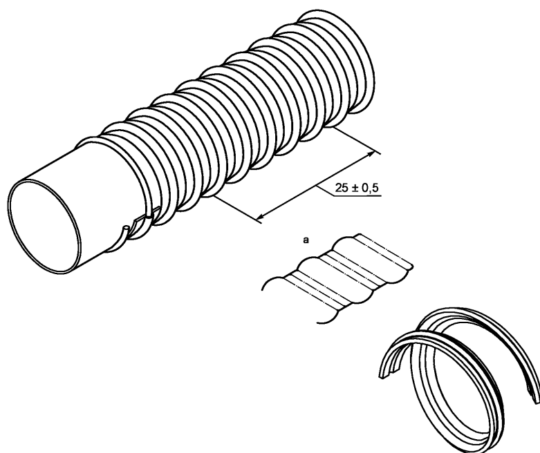
Рисунок 7 — Образец типа 7
