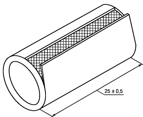
Рисунок 8 — Образец типа 8
