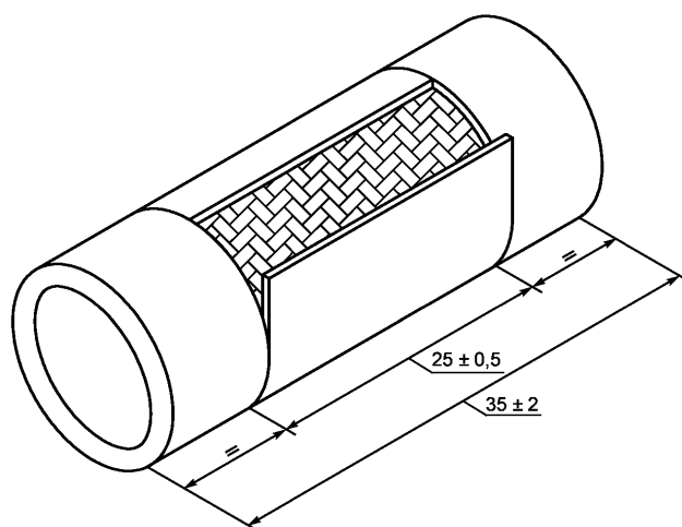
Рисунок 6 — Образец типа 6
