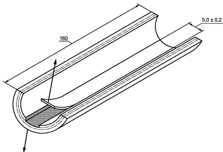
Рисунок 5 — Образец типа 5
