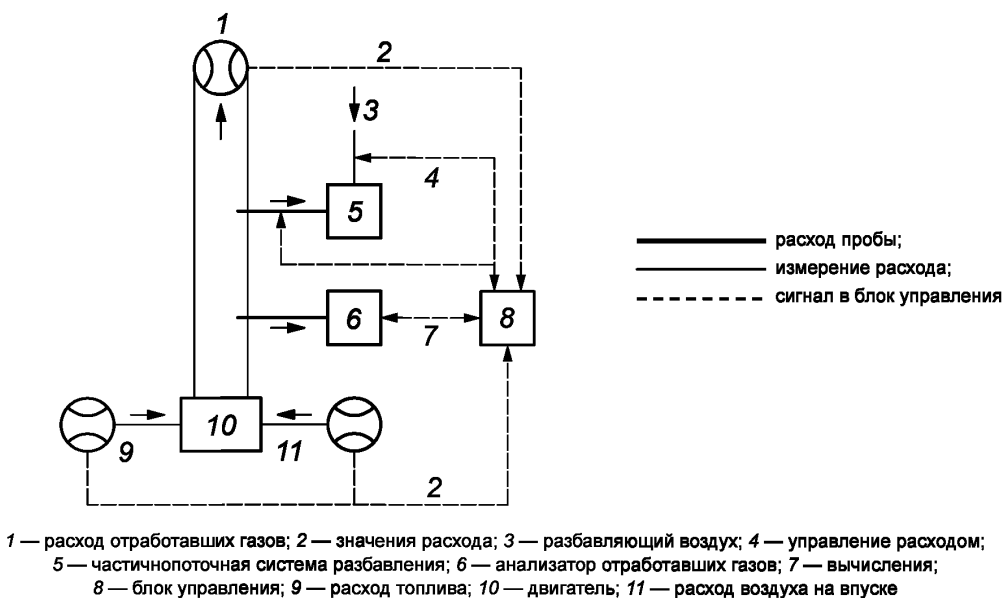
Рисунок 2 — Схема измерений в полнопоточной/частичнопоточной системах разбавления
