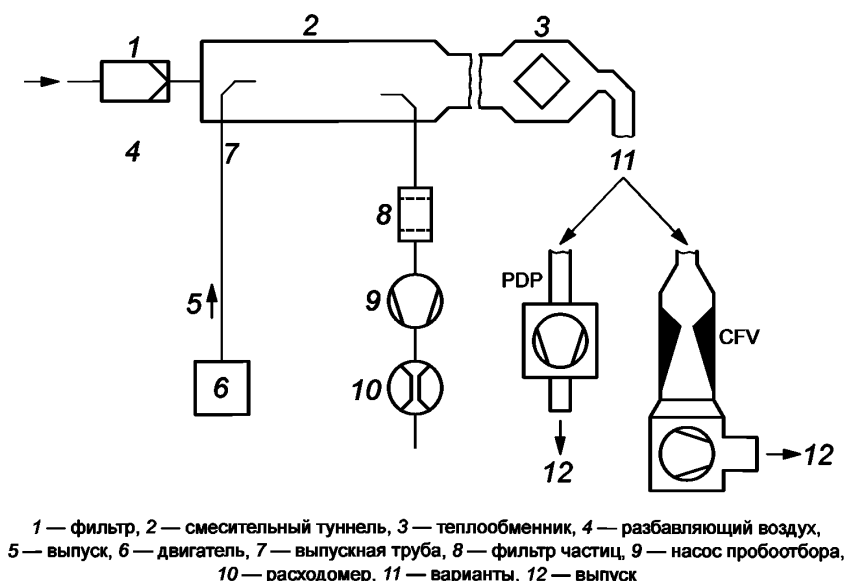
Рисунок 3 — Схема полнопоточной системы разбавления CVS
