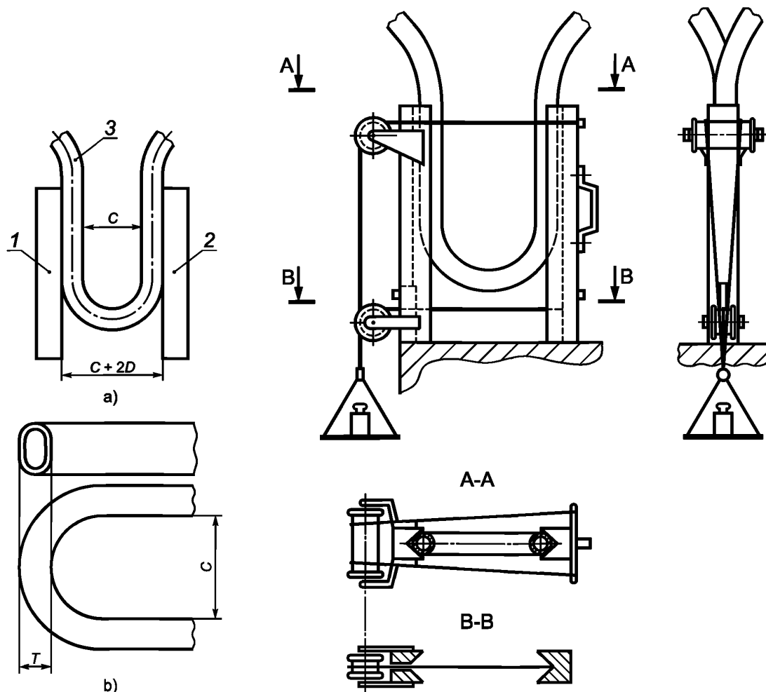
1 — направляющая А; 2 — направляющая В; 3 — испытуемый образец рукава
