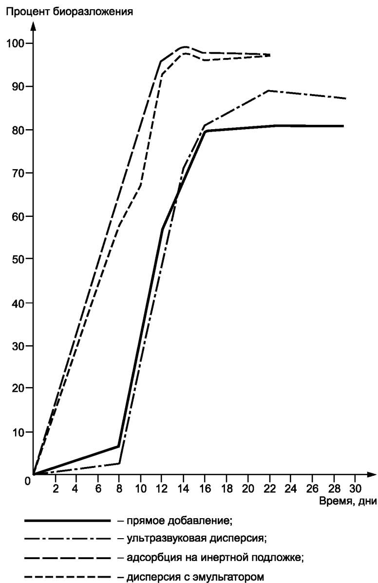
Рисунок А.1 — Кривые биоразлагаемости при использовании диизеокилфталата в качестве испытуемого соединения
