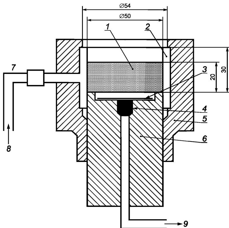
1 — испытуемый образец; 2 — резиновая трубка; 3 — пористая фильтровальная бумага; 4 — резиновая губка; 5 — подвижное зажимное устройство; 6 — стационарный поршень; 7 — пластиковый шланг; 8 — вход сжатого воздуха; 9 — система вакуума
