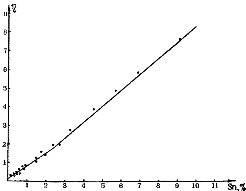
Рис.3. Эталонировочный график.
