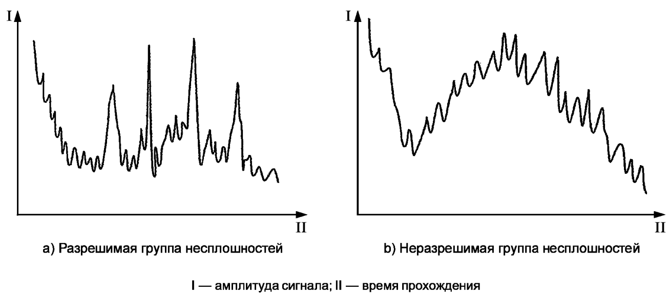
Рисунок 1 — Примеры сигналов с разверткой типа А из группы несплошностей в поковке или отливке
