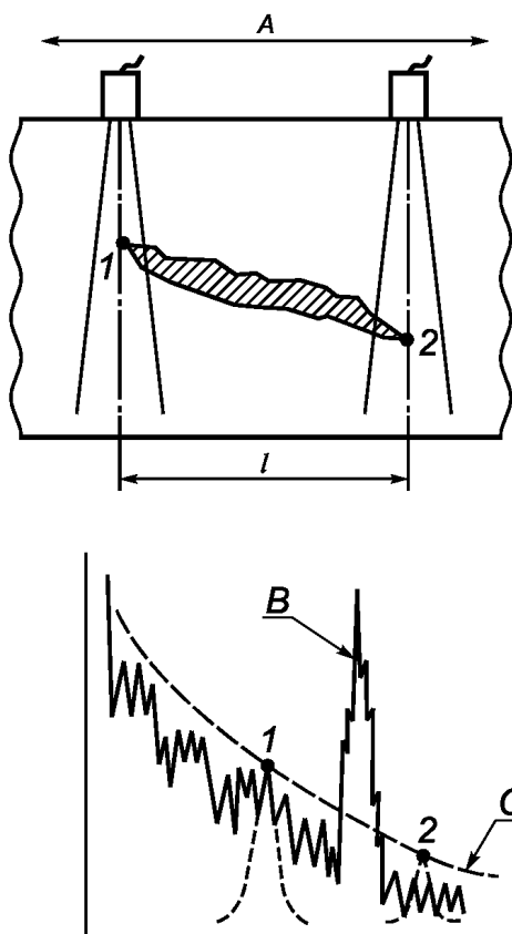
Рисунок D.4 — Метод падения амплитуды на 12 или 20 дБ от максимума
