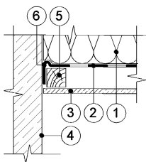
Рисунок 6.9 – Принципиальная схема примыкания к стене
