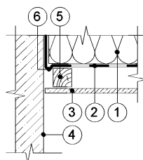
Рисунок 6.9 – Принципиальная схема примыкания к стене
