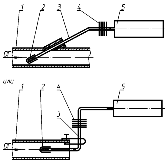
Рис. П12.6.1 Схема установки дымомера фильтрационного типа:
