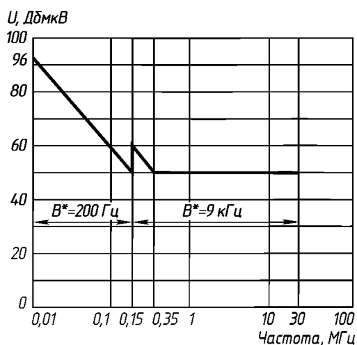
Рис. П15.14.2.2. Предельные уровни напряжений кондуктивных радиопомех на клеммах источников питания оборудования:
