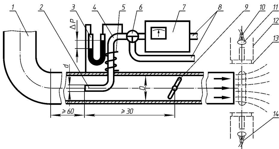
Рис. П12.5.1 Схема установки дымомера оптического типа:
