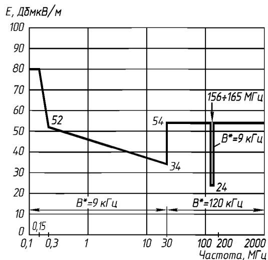
Рис. П15.14.2.3. Предельные уровни излучаемых помех от портов корпуса оборудования: B^* — ширина полосы пропускания измерительного приемника
