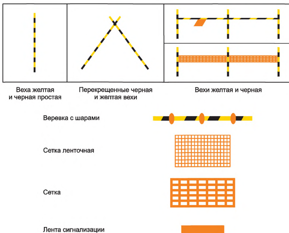
Рисунок Д.1 — Примеры сигнальных вех
