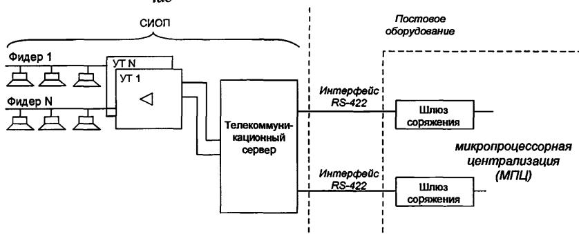
Рисунок 6.3 - Сопряжение МПЦ с ТКС
