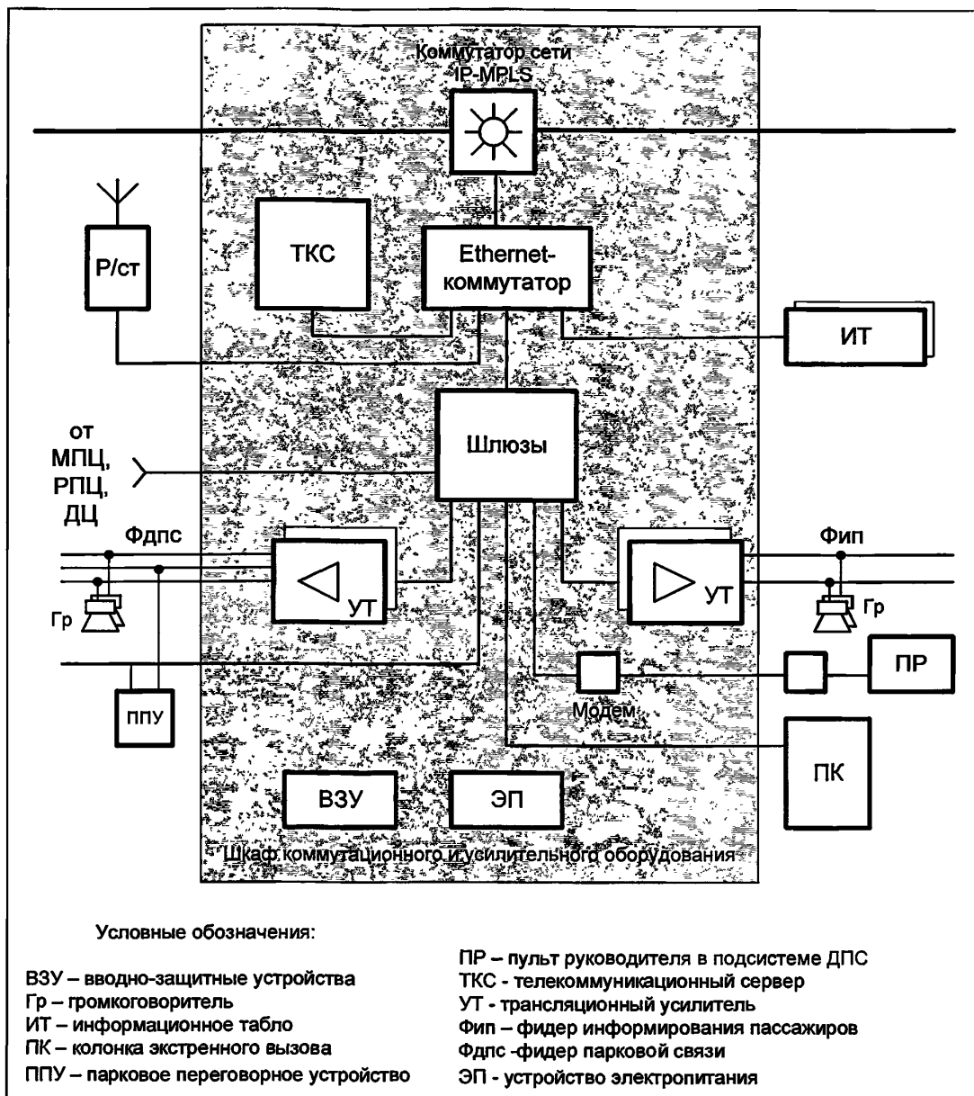
Рисунок 5.2 – Структурная схема СИОП на железнодорожной станции
