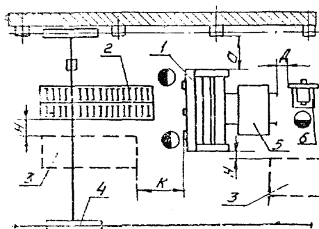
Ножницы кривошипные листовые с наклонными ножами (гильотинные)
