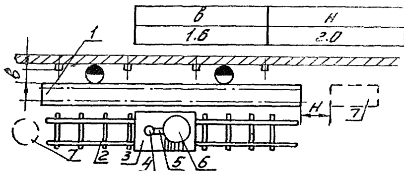
Установка электрошлаковой сварки
