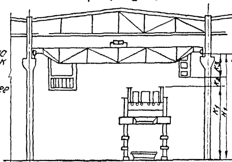
Пролеты, обслуживаемые мостовыми кранами
