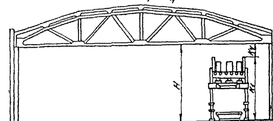
Пролеты, обслуживаемые мостовыми кранами
