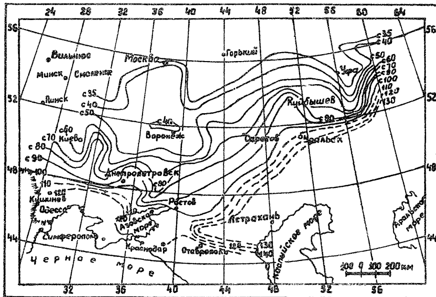
Карта изолиний коэффициентов вариаций весенне-го стока на территории степных и лесостепных районов Европейской части СССР.
