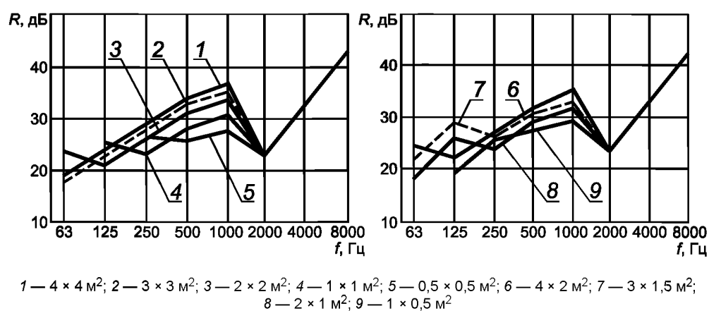
Рисунок 12 — Звукоизоляция пластины из органического стекла толщиной от 12 до 15 мм разных размеров
