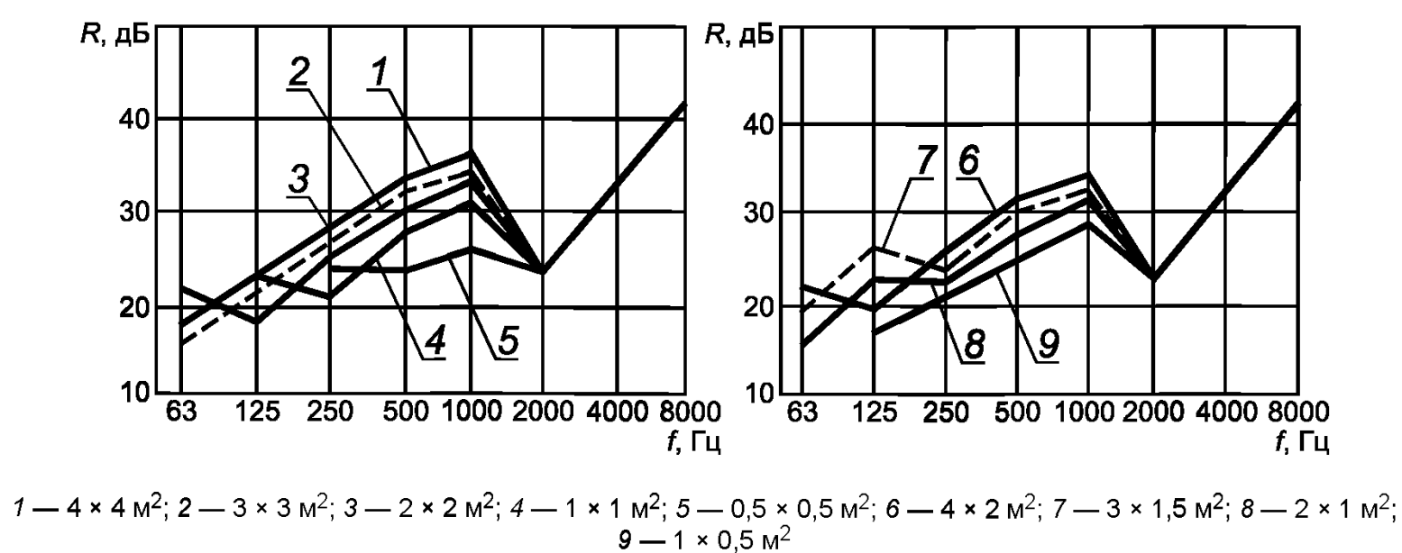
Рисунок 9 — Звукоизоляция пластин из алюминиево-магниевого сплава толщиной от 5 до 6 мм разных размеров
