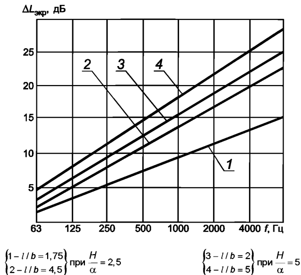
Рисунок 18 — Усредненные значения акустической эффективности экрана \Delta L_{\text{экр}}
