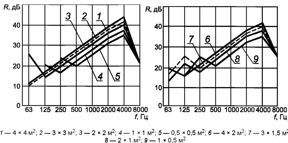
Рисунок 10 — Звукоизоляция пластин из органического стекла толщиной от 3 до 4 мм разных размеров
