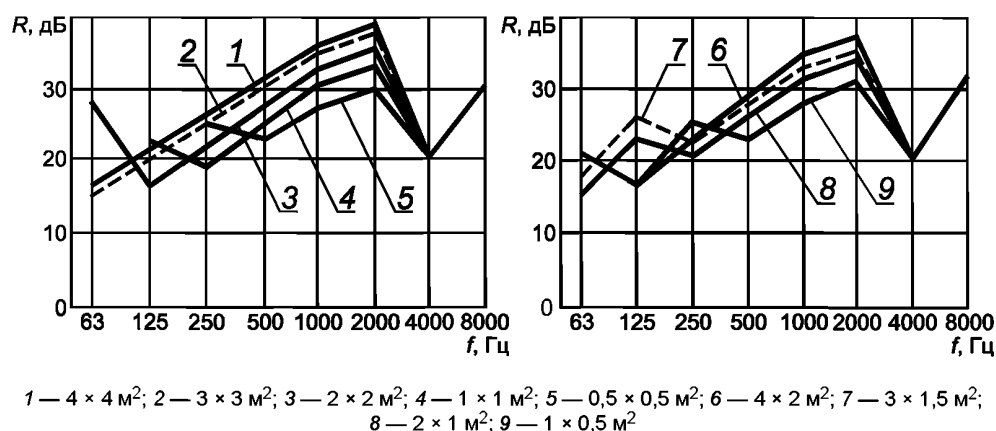
Рисунок 11 — Звукоизоляция пластины из органического стекла толщиной от 5 до 6 мм разных размеров
