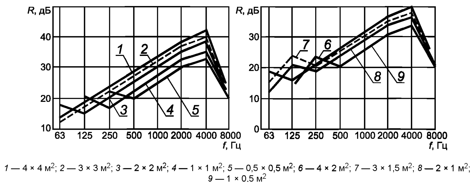
Рисунок 7 — Звукоизоляция пластин из алюминиево-магниевого сплава толщиной от 1,5 до 3 мм разных размеров
