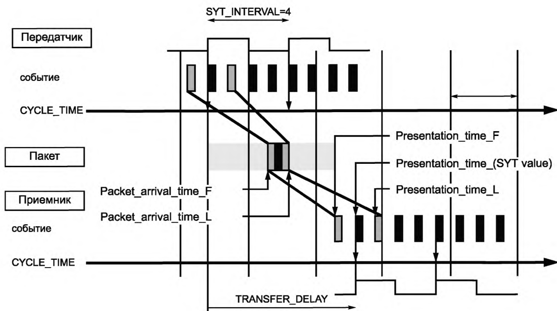
Рисунок 7 — Параметры передачи
