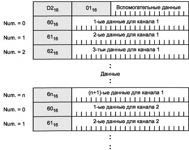
Рисунок 22 — Обобщенная последовательность квадлет высокой точности
