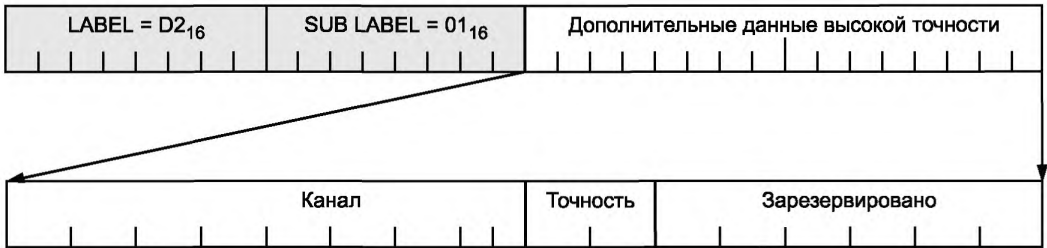
Рисунок 45 — Первые вспомогательные данные высокой точности
