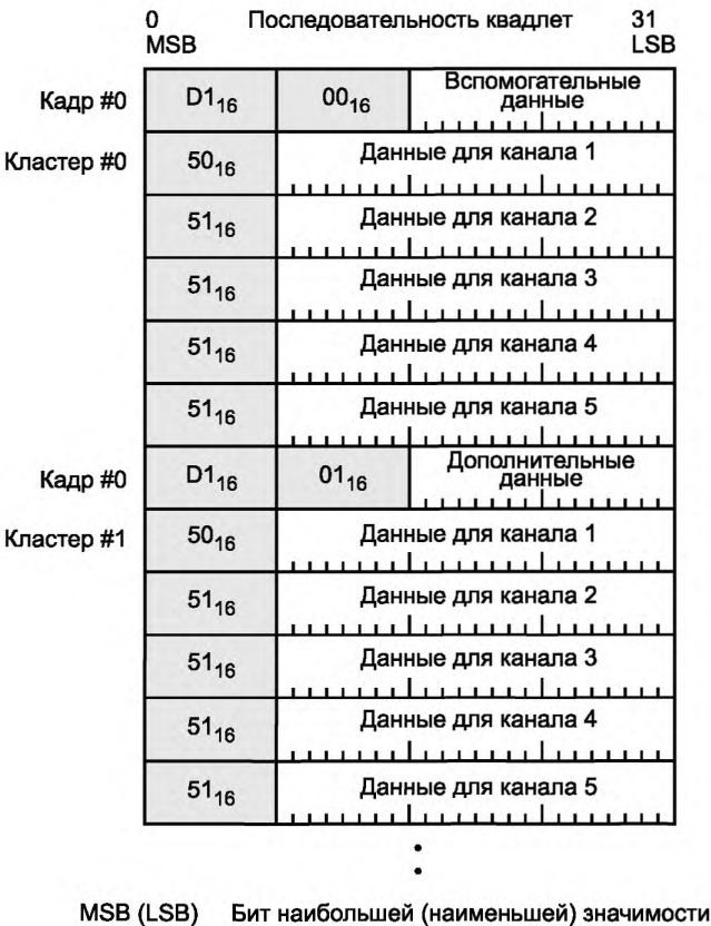
Рисунок 63 — Пример потока SACD в случае пяти каналов
