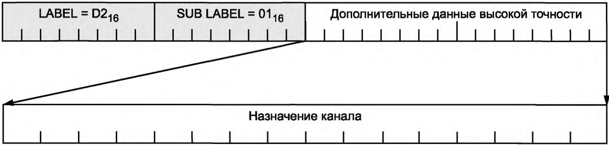
Рисунок 48 — Вспомогательные данные с назначением каналов высокой точности
