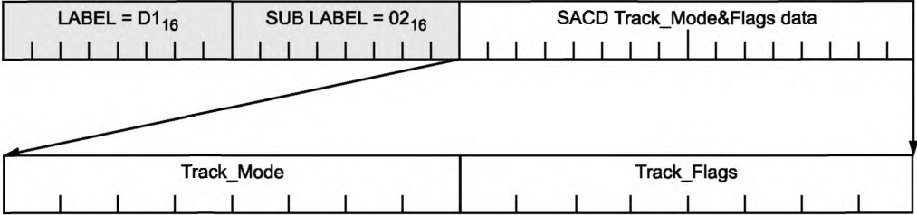
Рисунок 60 — Данные Track_Mode&Flags SACD
