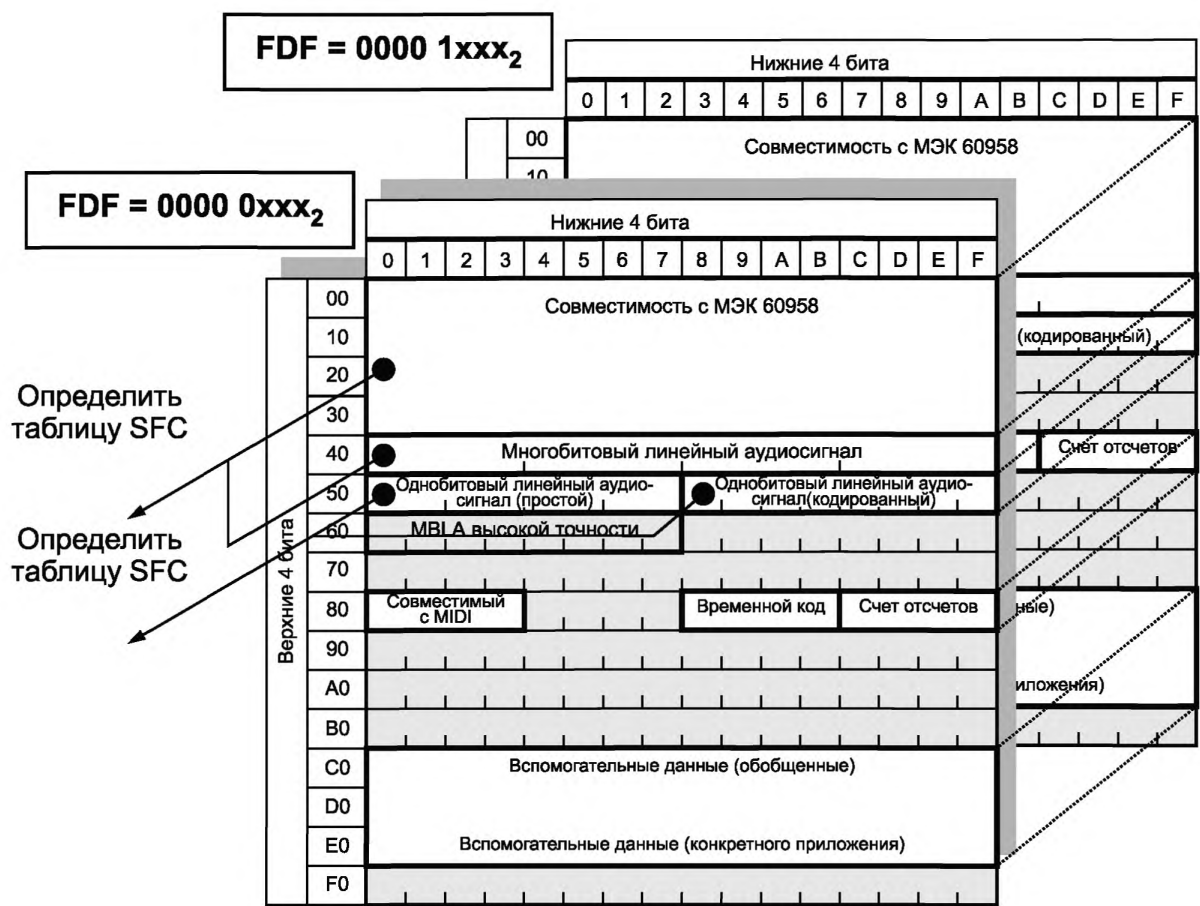
Рисунок 34 — FDF для AM824 и пространство LABEL AM824
