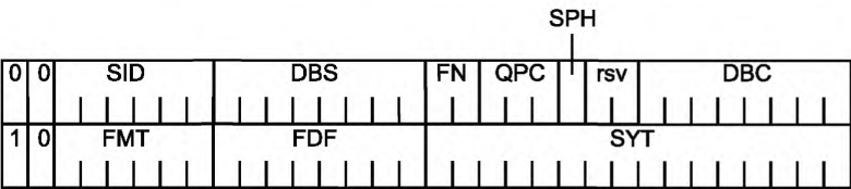
Рисунок 5 — Формат общего изохронного пакета (CIP)
