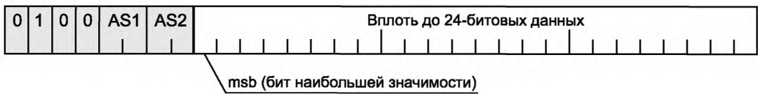
Рисунок 16 — Данные MBLA
