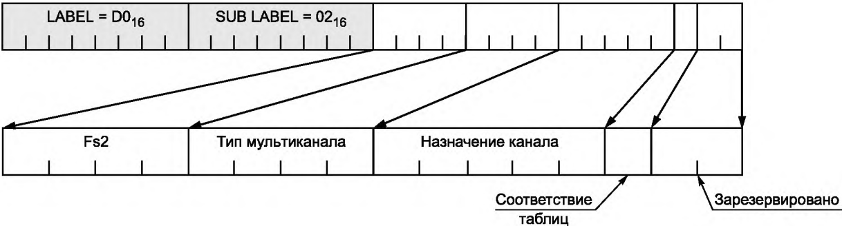
Рисунок 52 — Данные, передаваемые в точке начала данных
