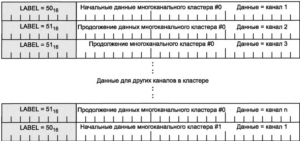
Рисунок 42 — Обобщенная последовательность квадлет однобитового аудиосигнала.
