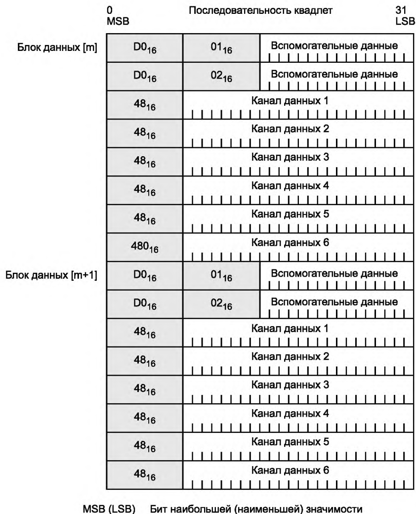
Рисунок 57 — Пример данных аудиосигнала DVD (DVD-Audio)
