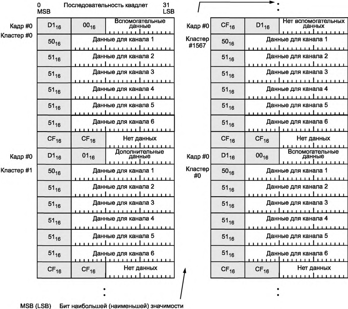
Рисунок 62 — Пример потока SACD в случае шести каналов
