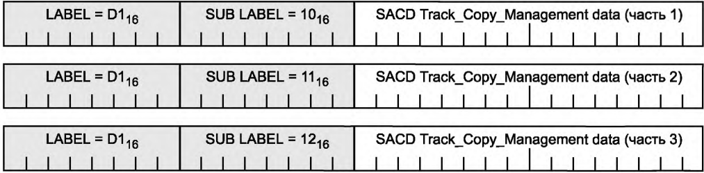
Рисунок 61 — Данные Track_Copy_Management SACD
