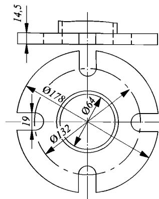
Рис. 5.1.18 Международное береговое соединение (судно)
