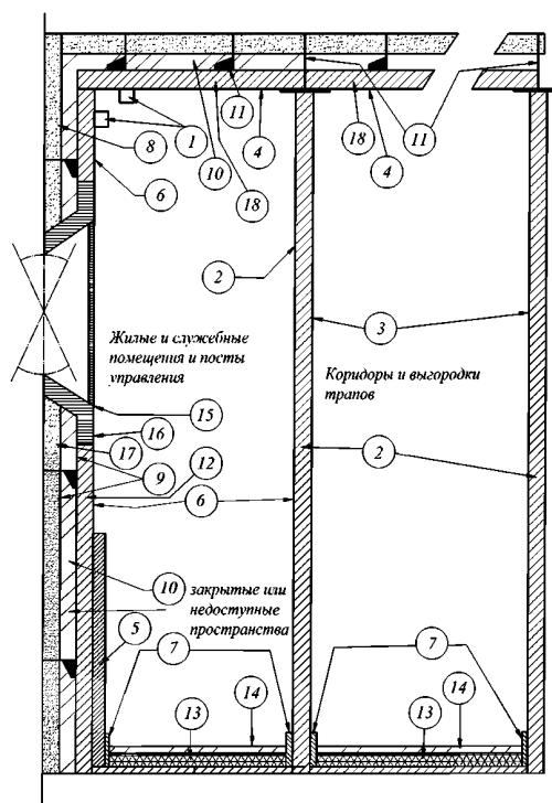
Рис. 2.3.10 Конструктивные элементы в жилых помещениях
