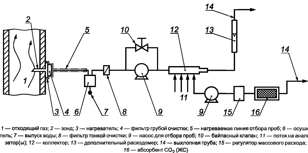
Рисунок 1 — Пример отбора проб для стационарных измерений
