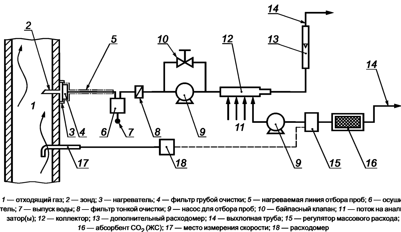
Рисунок 2 — Пример отбора пробы при пропорциональном отборе
