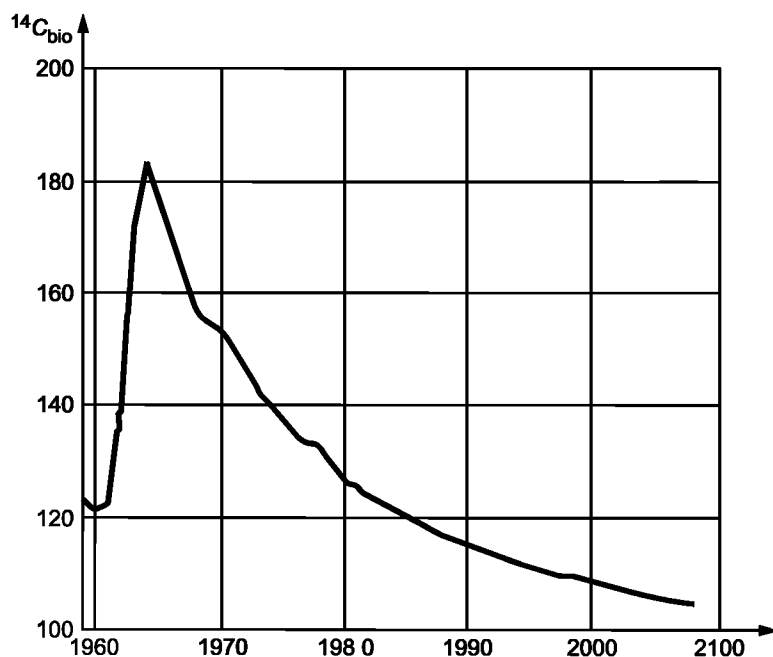
Рисунок Е.1 — Уменьшение значения ^{14}\text{C}_{\text{bioC}} в атмосферном воздухе с \text{CO}_2 (в pmC), измеренное на высокогорной альпийской станции в Вермунте (Австрия) и Jungfraujoch (Швейцария) (см. [14], для данных 2004—2008 гг. см. сообщение С. Пэлстры и И. Левина)
