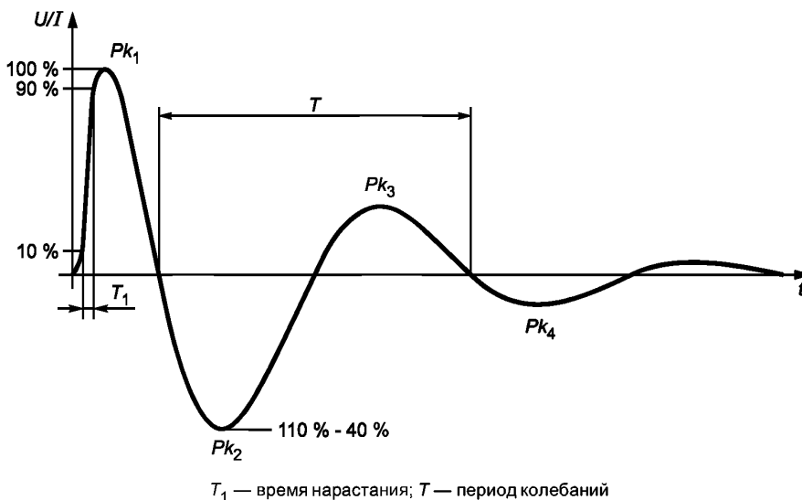
Рисунок 1 — Форма звонящей волны (напряжение холостого хода и ток короткого замыкания)
