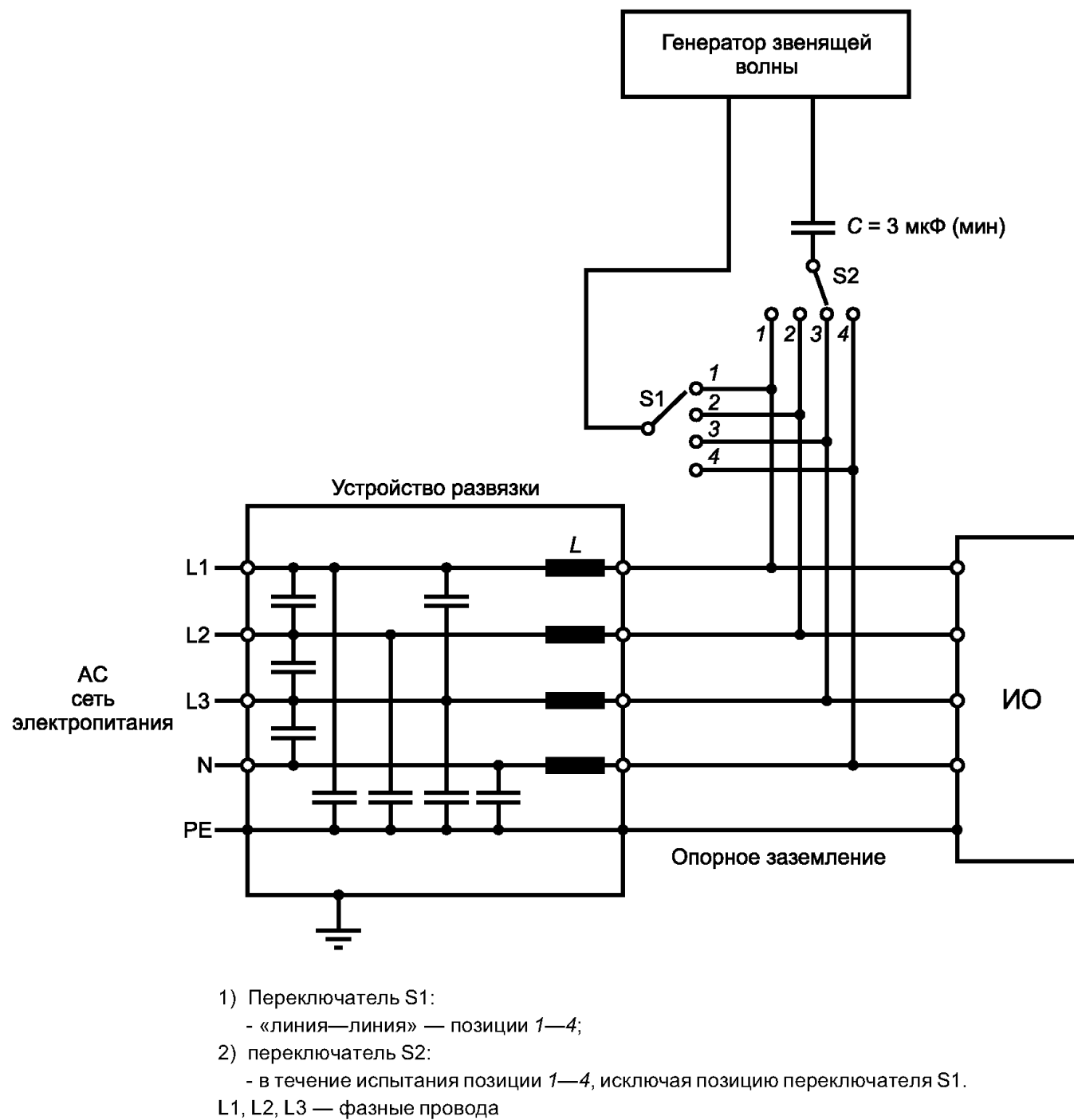
Рисунок 7 — Пример испытательной установки для линий переменного тока (трехфазная сеть), емкостная связь «линия L3—линия L1»
