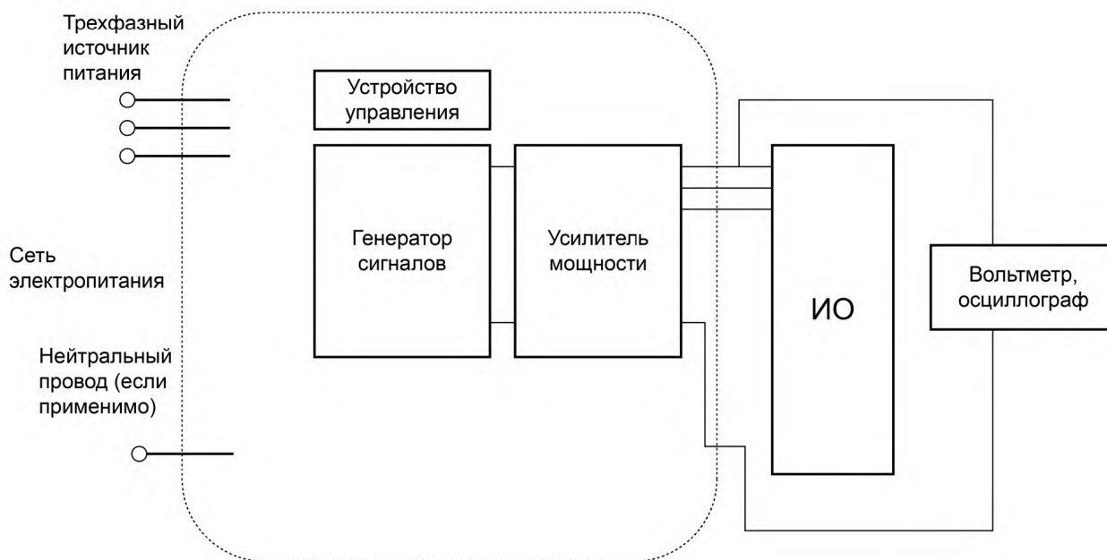
Рисунок 3 — Схема устройства испытательной установки для создания несимметричных напряжений
