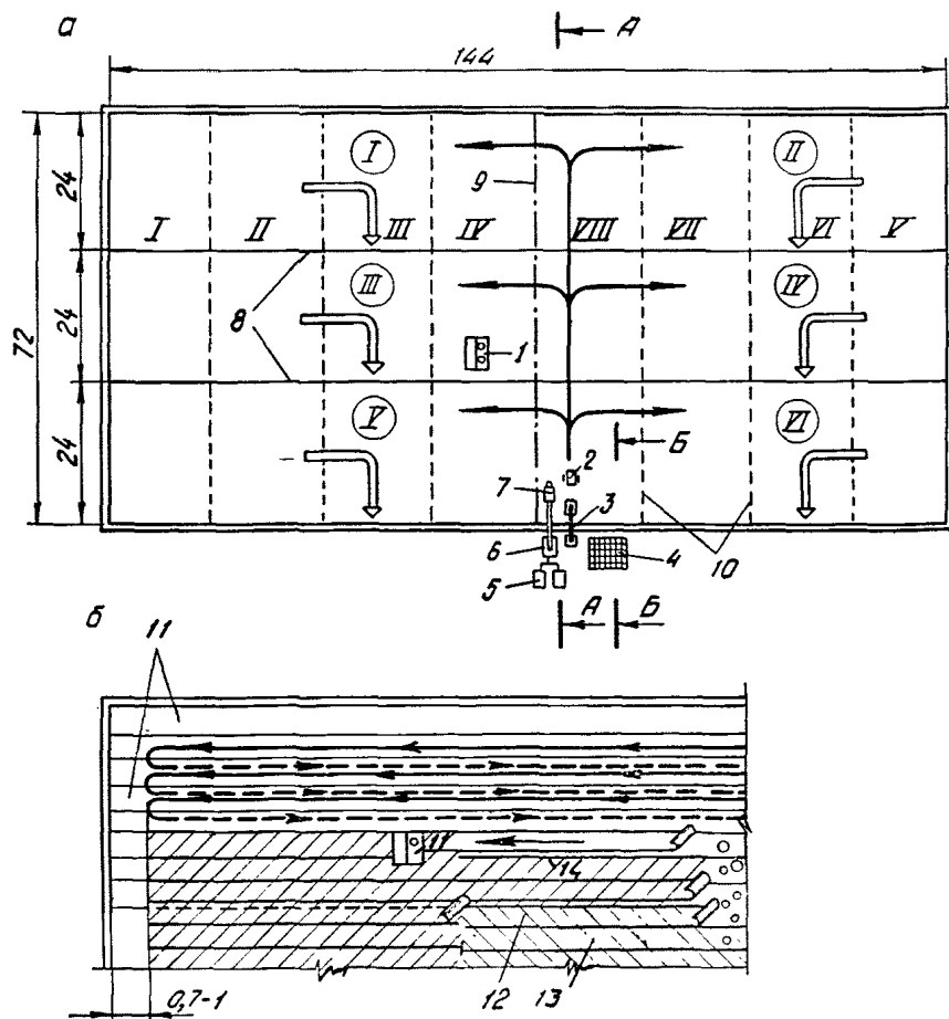
Рис. Схема организации работ на строительстве корпуса (а) и схема производства работ на делянке (б)
