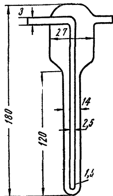
Рис. 5. Поглотительный прибор Зайцева.
