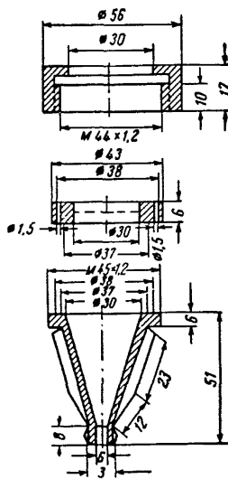
Рис. 4. Плексигласовый патрон.
