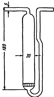
Рис. 5. Погло- тельный прибор с пористой пластин- кой.
