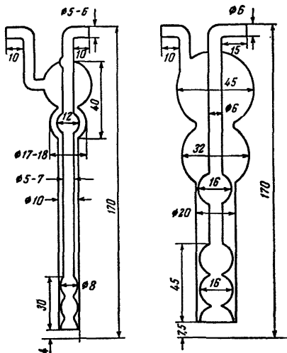
Рис. 6. Погло- тельные приборы Рыхтера.
