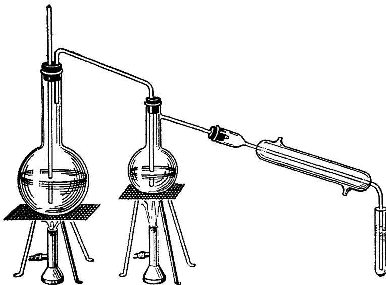
Рис. 13. Прибор для перегонки с водяным паром
