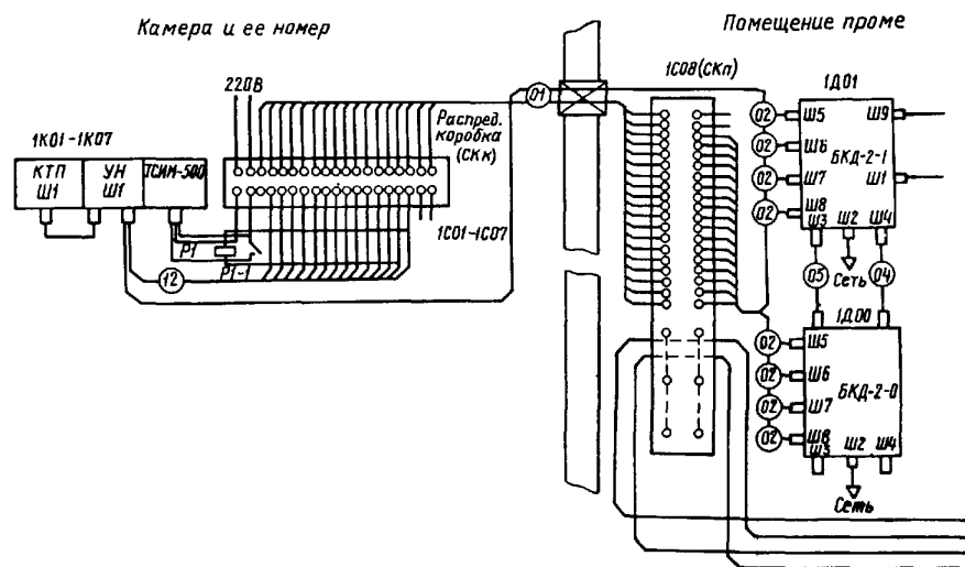
Рис.6. Принципиальная электрическая схема
