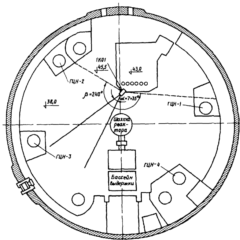
Рис.7. Схема установки КТП в центральном зале:
