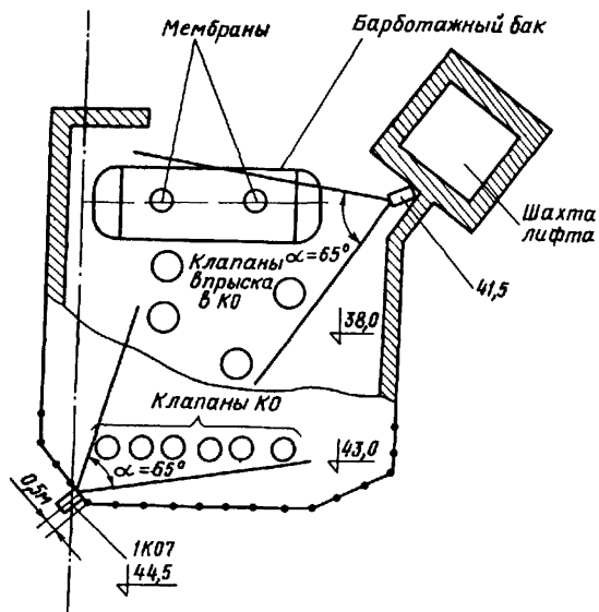
Рис.9. Схема установки КТП у клапанов К0 и барботажного бака
