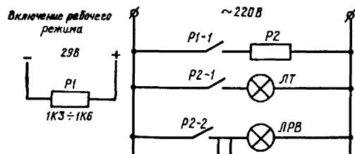
Рис.10. Схема освещения палубы ПЦН:
