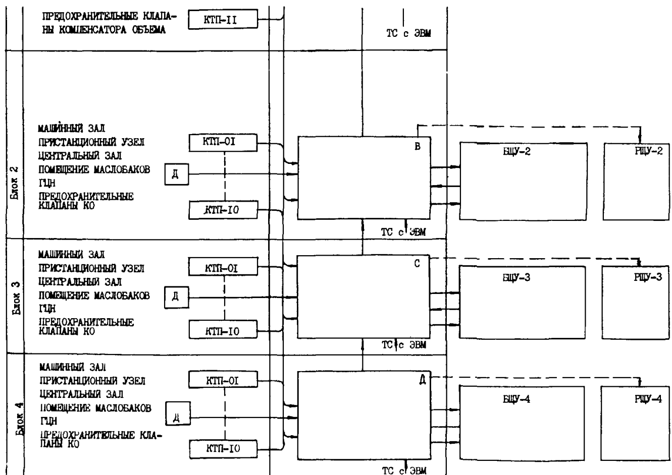
Рис.5. Структурная схема телевизионных каналов комплекса ДВК на АЭС с блоками ВВЗФ-1000
