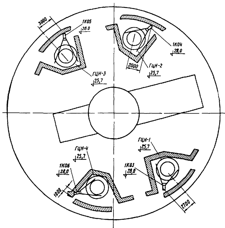
Рис.8. Схема установки КТП в боксе ГЦН:
