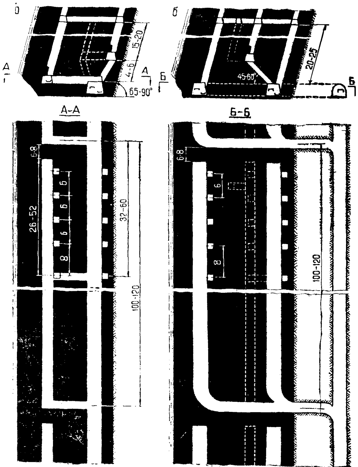
Рис. 2. Подготовка выемочных блоков на откаточном горизонте при групповой (а) и полевой (б) схемах вскрытия одиночного пласта
