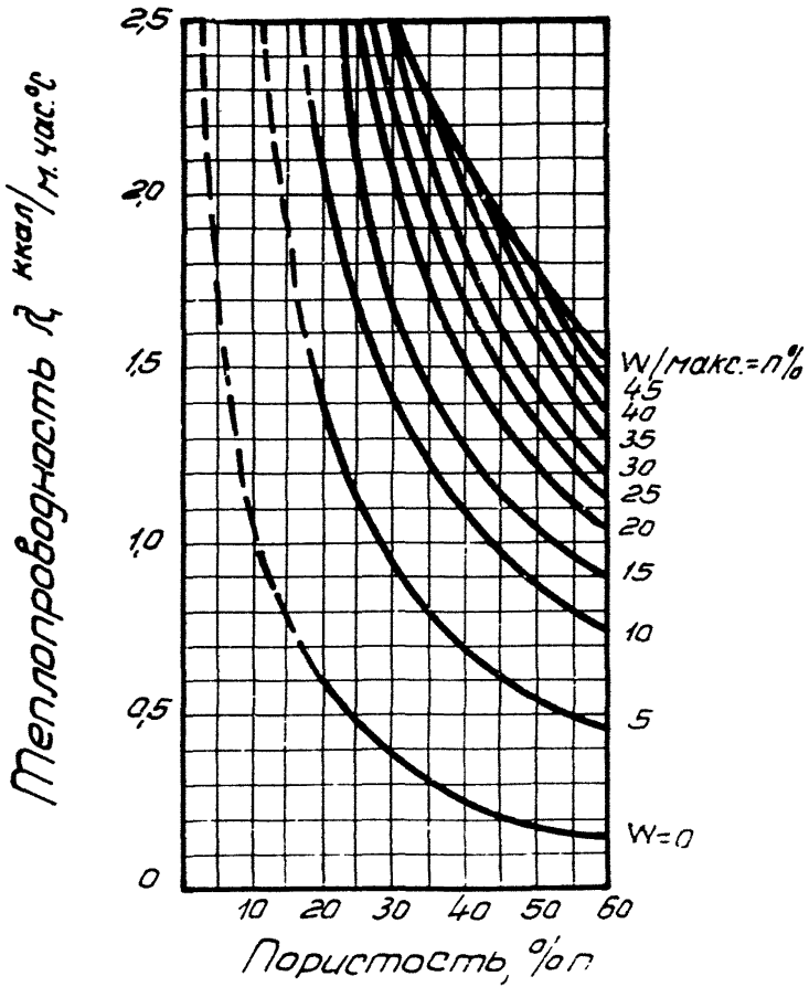
Рис. 6. Графики значений коэффициента теплопроводности чистого песка в функции объемной влажности и пористости (при t = +20^\circ\text{С} )
