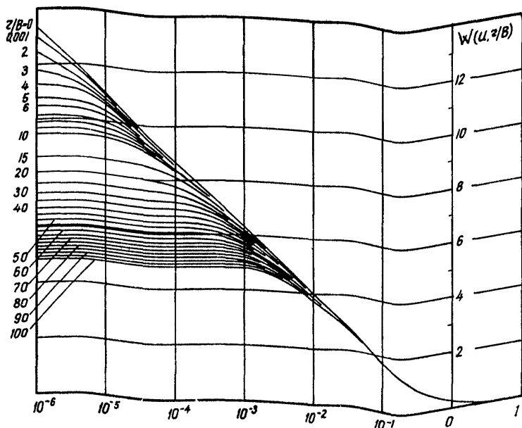
Рис. 15. График функции W(u, z/B) .
