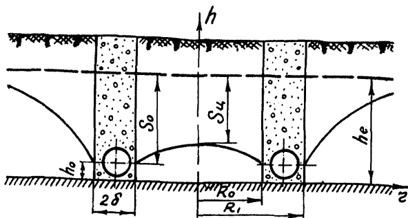
Рис. 11. Схема к расчету кольцевого горизонтального дренажа совершенного типа.
