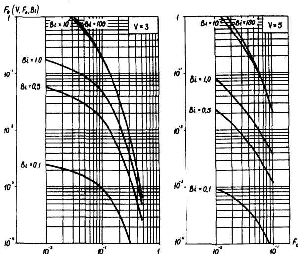
Рис. 18. График функции \bar{z}(v, f_0, B_i) .
