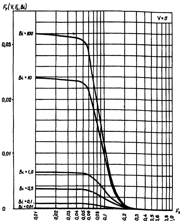
Рис. 17. График функции \mathcal{F}_7(v, f_0, B_i) .
