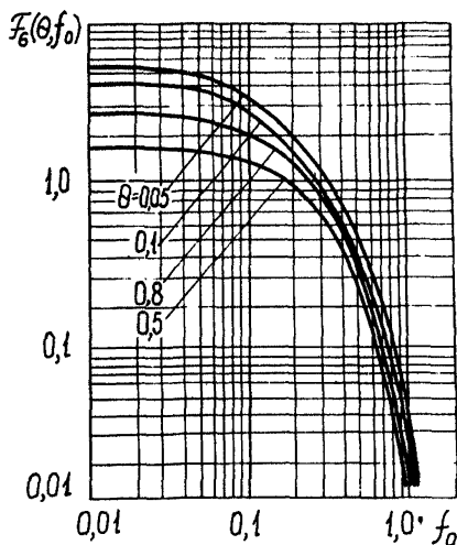
Рис. 13. График функции F_6(\theta, f_0) .
