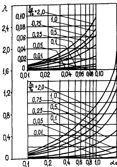
Рис. 6. График для определения величины \lambda .
