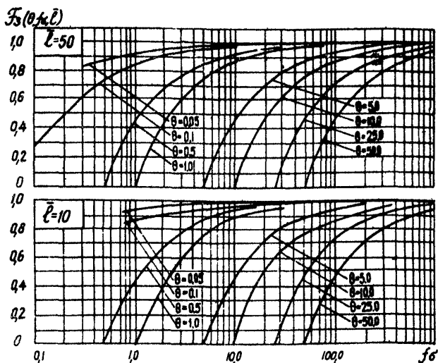
Рис.8. График функции F_3(\theta, f_\beta, \bar{l}) .
