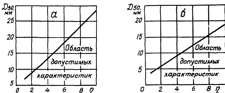
Рис.21. График для подбора первого слоя обсыпки:
