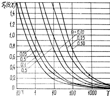
Рис. 4. График функции \mathcal{F}_2(\theta, \gamma) .
