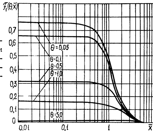
Рис. 3. График функции \mathcal{F}_1(\theta, \bar{x}) .
