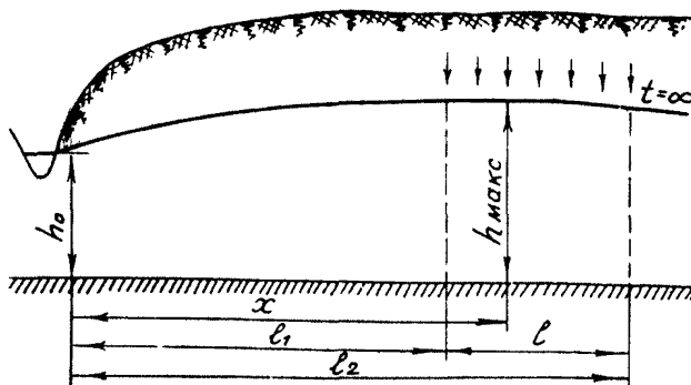
Рис.23. Схема к расчету повышения уровня грунтовых вод во времени при усиленной инфильтрации на полосе, вытянутой вдоль дрена.
