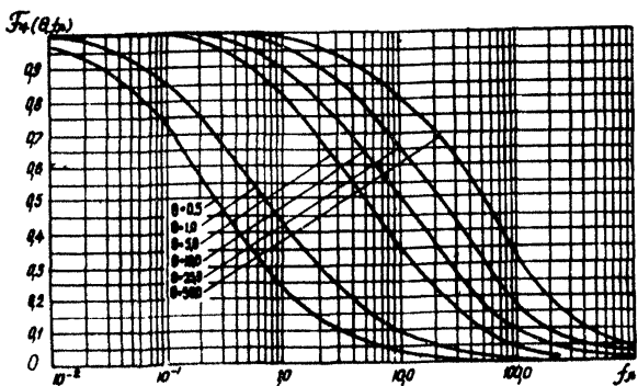
Рис. 9. График функции F_4(\theta, f_0) .
