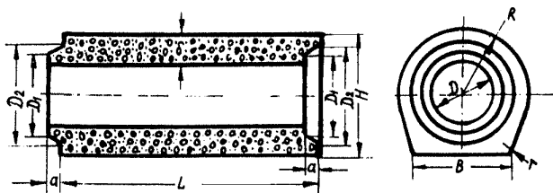
Рис. 1. Схема дренажного трубофилтра.
