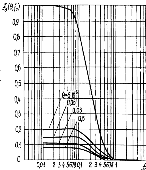
Рис. 12. График функции \mathcal{F}_5(\theta, f_0) .
