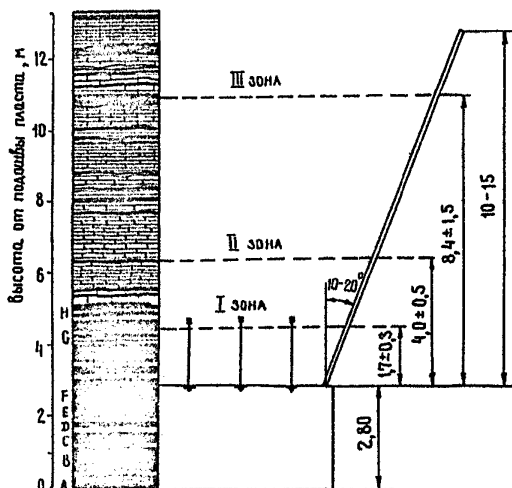
Рис. 2. Схема расположения горизонтальных водопрводящих зон в породах кровли выработок (I, II и III) и дренажной скважины
