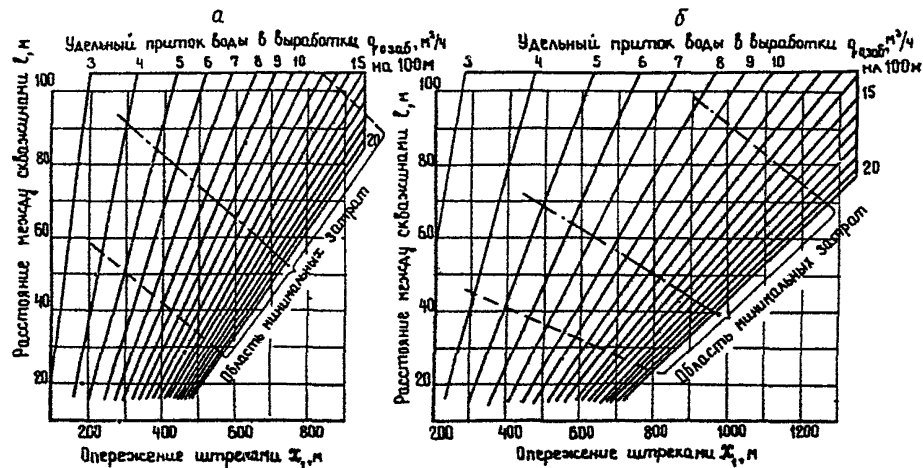
Рис. 3. Номограммы для определения расстояния между скважинами l в зависимости от опережения панельными штреками Z и степени обводненности пород q_{\text{об}} при допустимой величине удельного притока воды в выемочные блоки q_{\text{доп}} = 2 \text{ м}^3/\text{ч} на 100 м:
