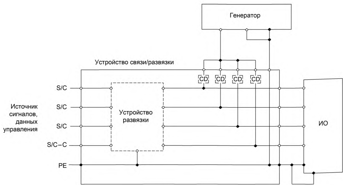
Рисунок 8b — Испытательная установка, снабженная специальными заземляющими проводниками
