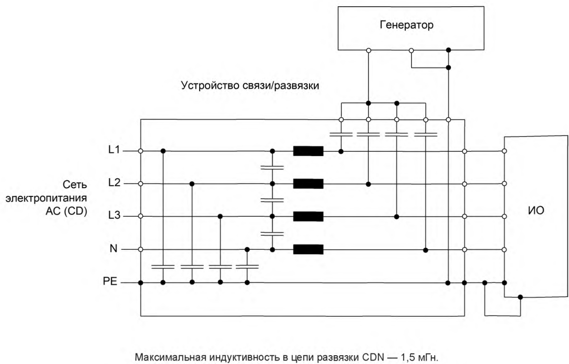
Рисунок 6b — Испытательная установка, снабженная специальными заземляющими проводниками
