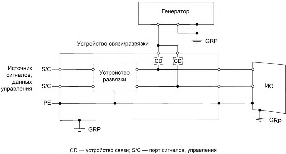
Рисунок 7a — Испытательная установка, снабженная опорной пластиной заземления (GRP)
