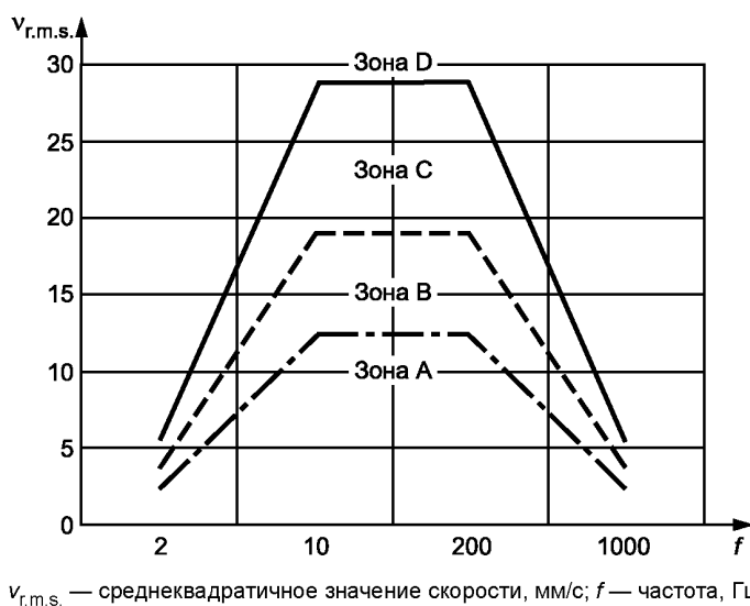
Рисунок В.10 — Границы зон для вибрации трубопроводов и гасителей пульсаций компрессора с вертикальным расположением цилиндров
