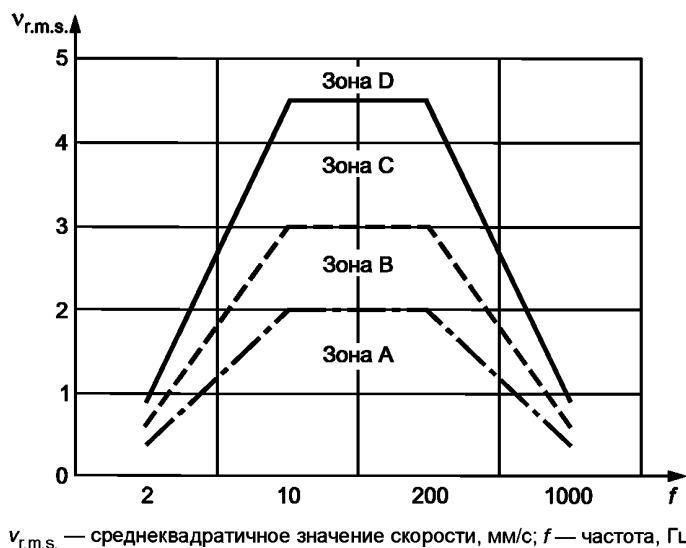
Рисунок В.1 — Границы зон для вибрации фундамента компрессора с горизонтальным расположением цилиндров
