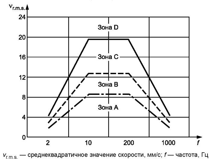
Рисунок В.9 — Границы зон для продольной вибрации цилиндров компрессора с вертикальным расположением цилиндров
