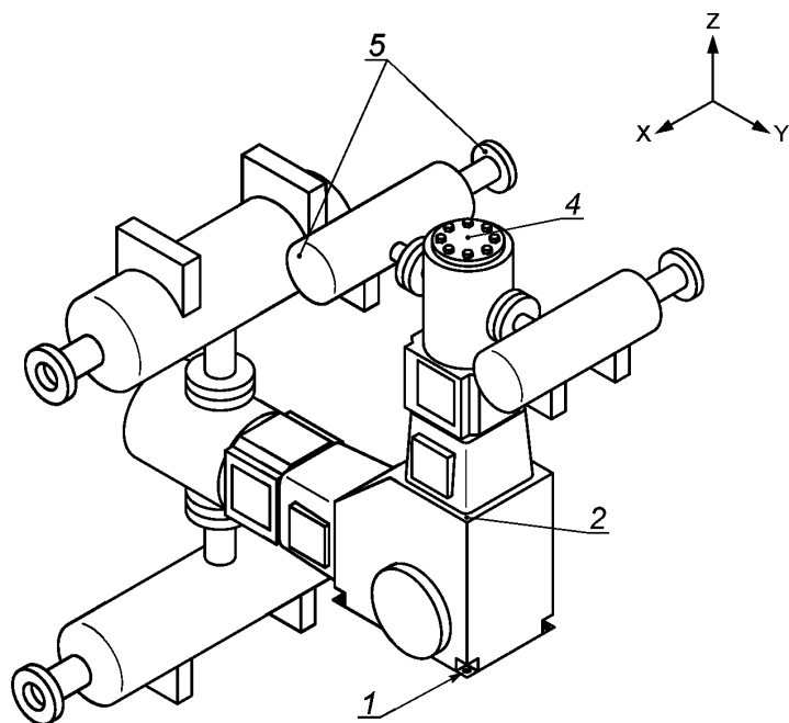
1 — болтовое крепление; 2 — угол корпуса; 3 — точка между цилиндрами (если число цилиндров более двух); 4 — фланец цилиндра; 5 — устройство выравнивания пульсаций
