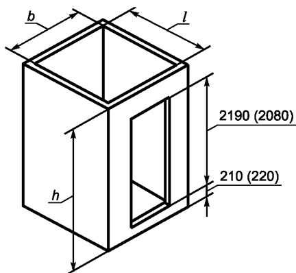
Средний блок
