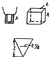
Рис. 17. К расчету растворимости металла в ртути.
