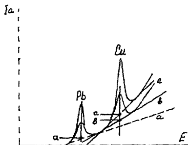
Рис. 11. Способы измерения высот анодных пиков от касательных:
