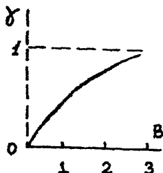
Рис. 7. Зависимость степени истощения ( \gamma ) от условия электролиза ( B )
